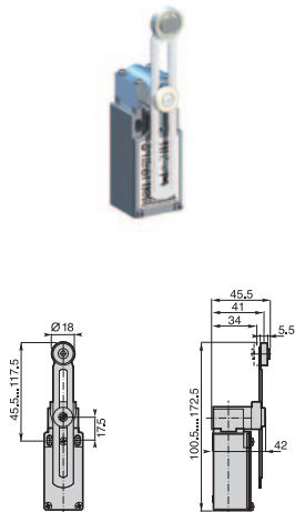
Min. actuating torque 0,10Nm (0,32Nm) ⇄ Weight 255 g
