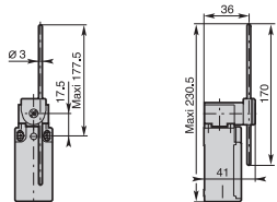
Min. actuating torque 0,10Nm (0,32Nm ⇨) Weight 105 g
