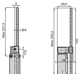
Min. actuating torque 0,10Nm (0,32Nm ⇨) Weight 115 g
