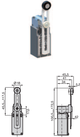
Min. actuating torque 0,10Nm (0,32Nm) ⇄ Weight 250 g
