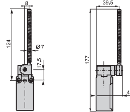
Min. actuating torque 0,10Nm Weight 105 g
