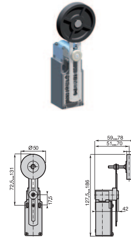
Min. actuating torque 0,10Nm (0,32Nm) ⇄ Weight 265 g
