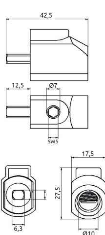
SR 50 (IP20)
