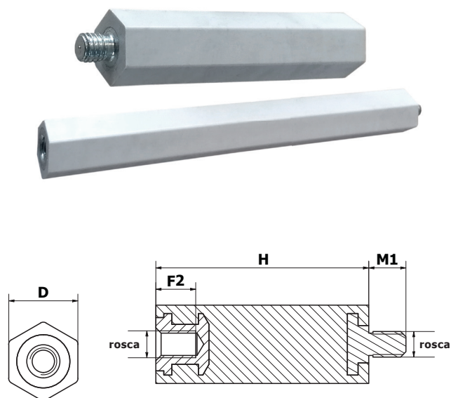
Dimensões (mm)
