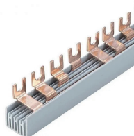
Barramentos MCB de 1 m
