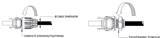
Especificação de montagem
