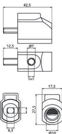
SR 50 (IP20)
