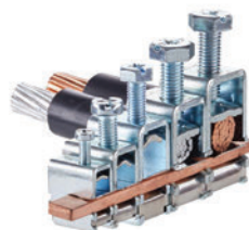
Zaciski szynowe MAE
