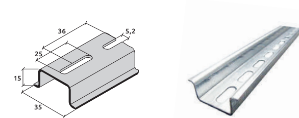
TS 35 x 15 perforovaná (5,2 x 25 mm) Zn
