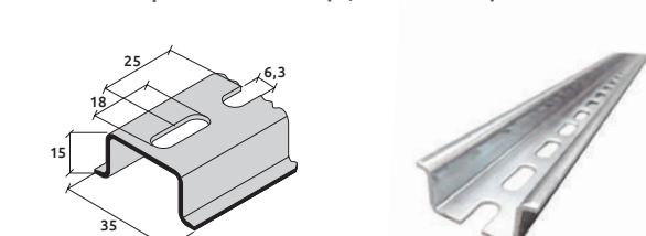
TS 35 x 15 perforovaná (6,3 x 18 mm) Zn
