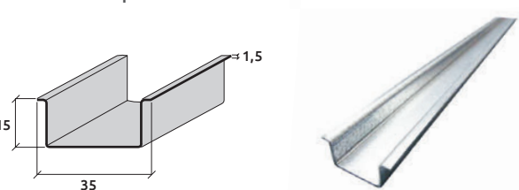
TS 35 x 15 plná Zn
