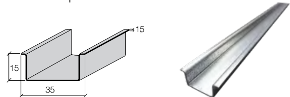
TS 35 x 15 plná
