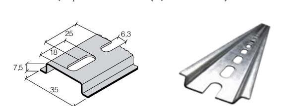
TS 35 x 7,5 perforovaná (6,3 x 18 mm)
