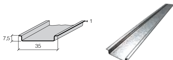
TS 35 x 7,5 plná
