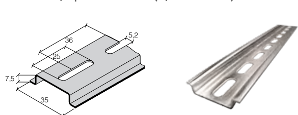
TS 35 x 7,5 perforovaná (5,2 x 25 mm)
