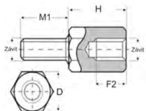
Rozměry (mm)
