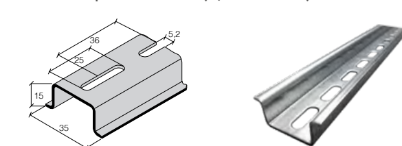
TS 35 x 15 perforovaná (5,2 x 25 mm)
