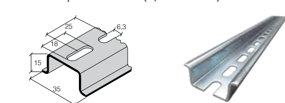
TS 35 x 15 perforovaná (6,3 x 18 mm)
