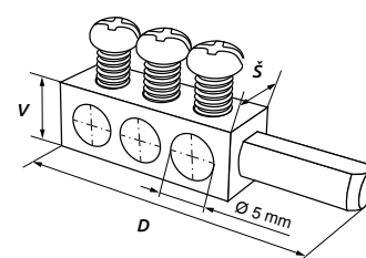
Svorkovnice MPIN
